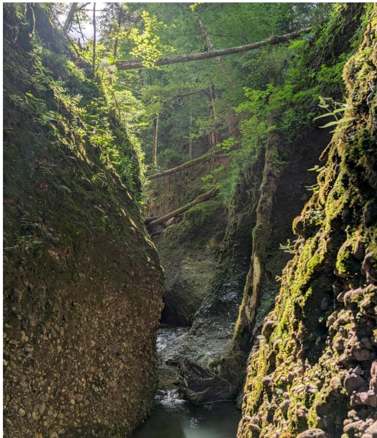
Abbildung: Um Verklausugen und Rutschungen im Gerinne zu verhindern, müssen Gefahrenträger wie hier im Prässerebach entfernt werden.
